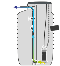
Conduite de sortie en polyéthylène (évacuation des eaux usées)
