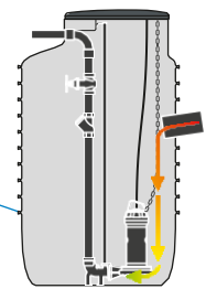
Prééquipement pour conduite d' entrée (entrée des eaux usées)
