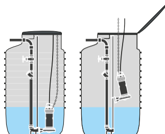
Dispositif d'accouplement au fond (DAC) qui permet de remplacer rapidement la pompe même lorsque le réservoir est plein
